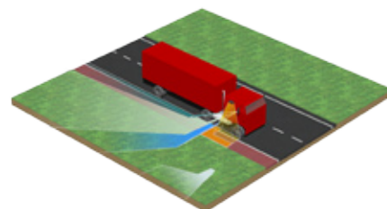
Huidig zichtveld Europese regeling, zonder DOBLI®
